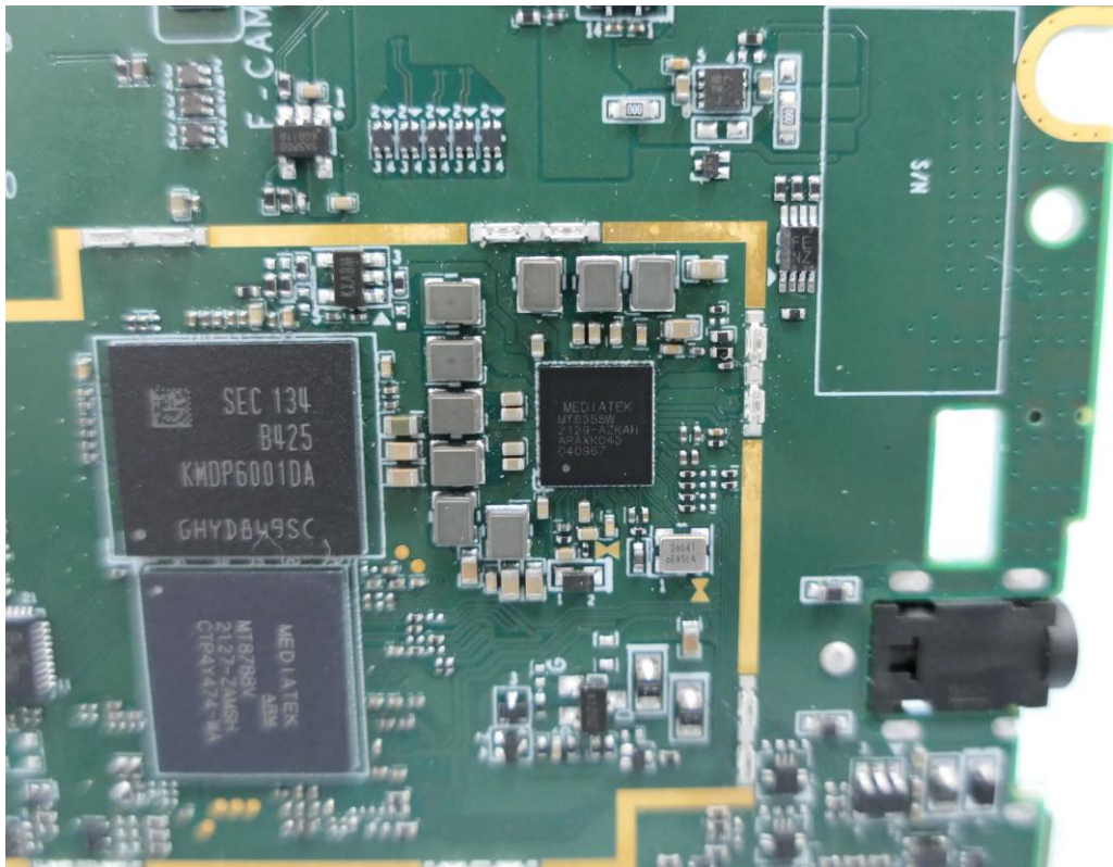
( 24 ) EUT Photo
