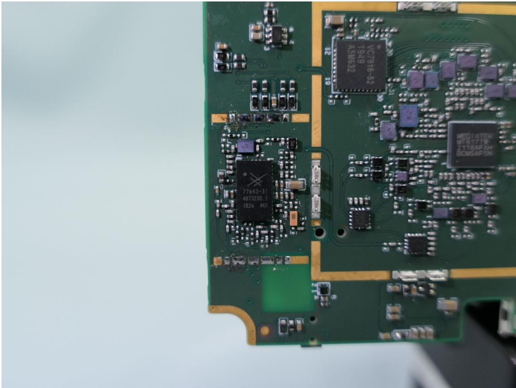
( 27 ) EUT Photo
