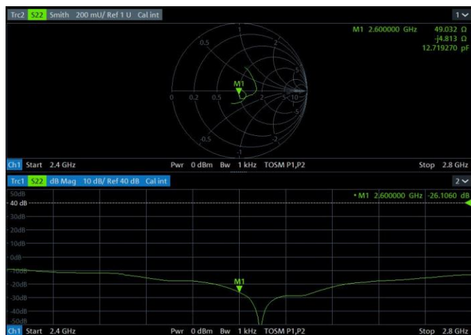
D2600V2_1005
