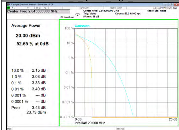
B41_1_Q16_High_
