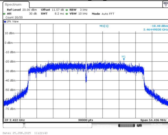
11AX40MIMO_Ant2_2452
