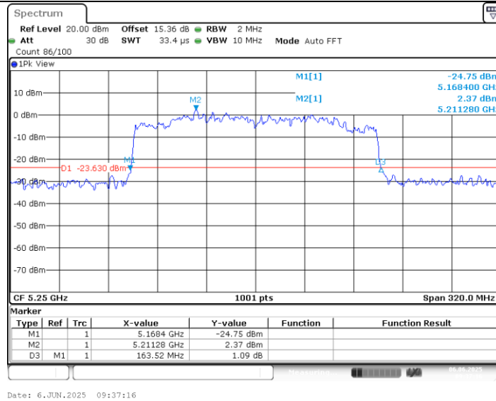
11AX160MIMO_Ant2_5250
