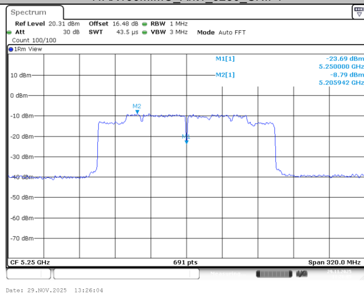
11AX160MIMO_Ant2_5250_UNII-1
