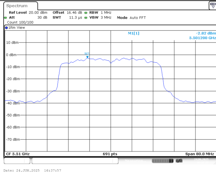
11AX40MIMO_Ant2_5510
