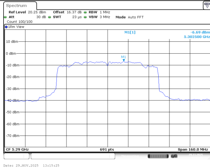
11AX80MIMO_Ant2_5290
