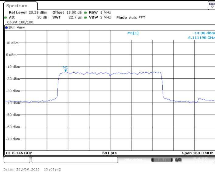
11AX80MIMO_Ant2_6145
