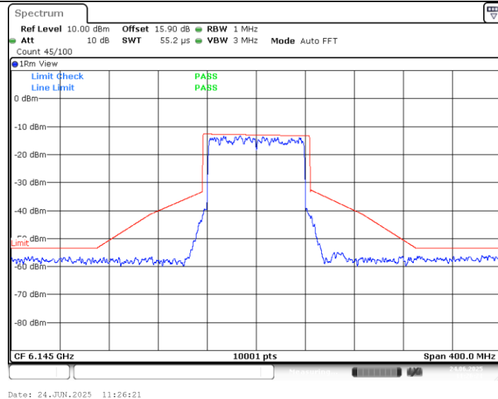
11AX80MIMO_Ant2_6145
