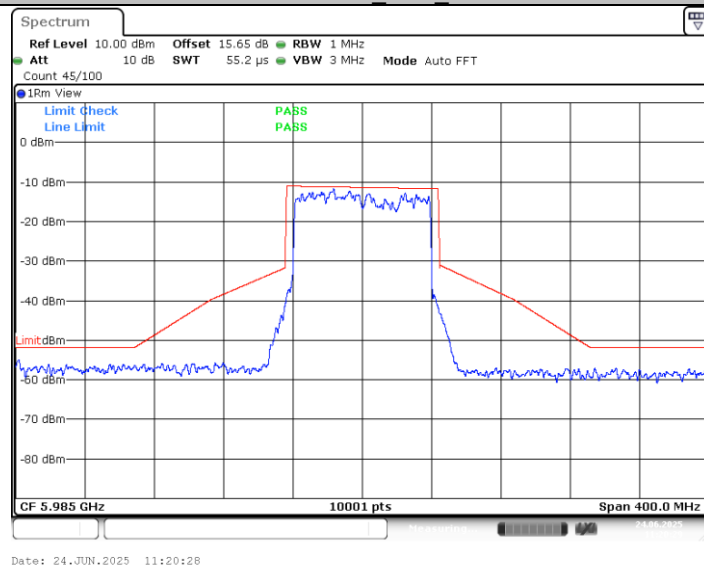
11AX80MIMO_Ant2_5985
