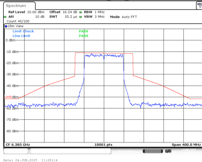
11AX80MIMO_Ant2_6385
