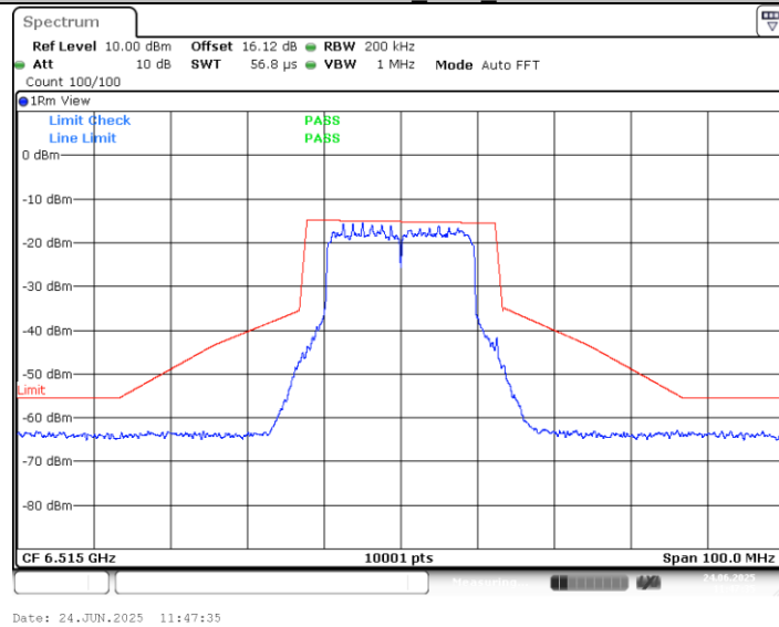
11AX20MIMO_Ant2_6515
