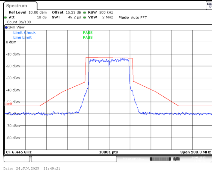
11AX40MIMO_Ant2_6445
