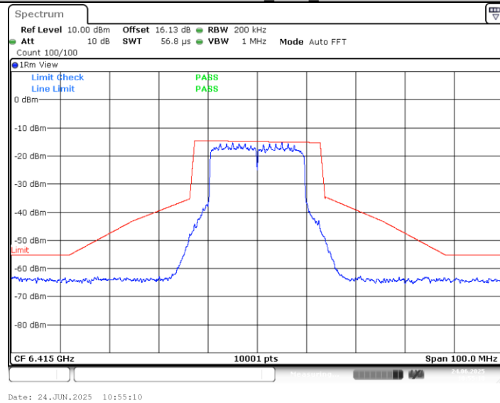
11AX20MIMO_Ant2_6415
