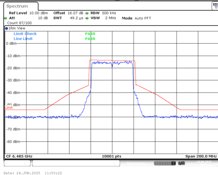
11AX40MIMO_Ant2_6485
