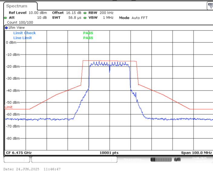
11AX20MIMO_Ant2_6475
