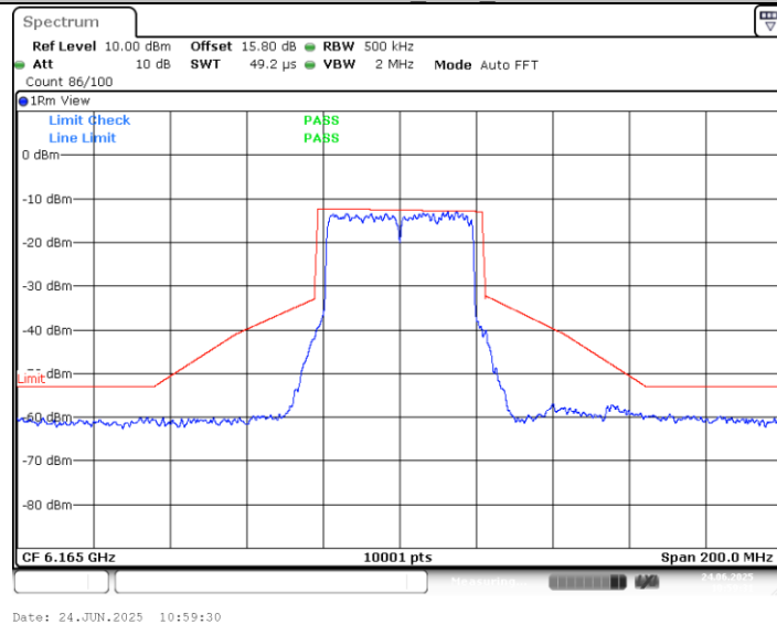
11AX40MIMO_Ant2_6165
