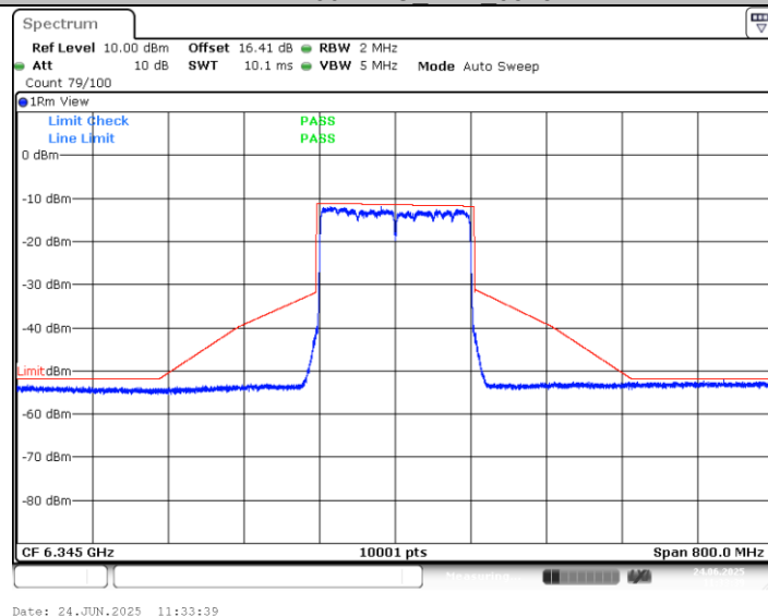
11AX160MIMO_Ant2_6345
