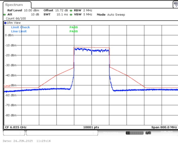
11AX160MIMO_Ant2_6025
