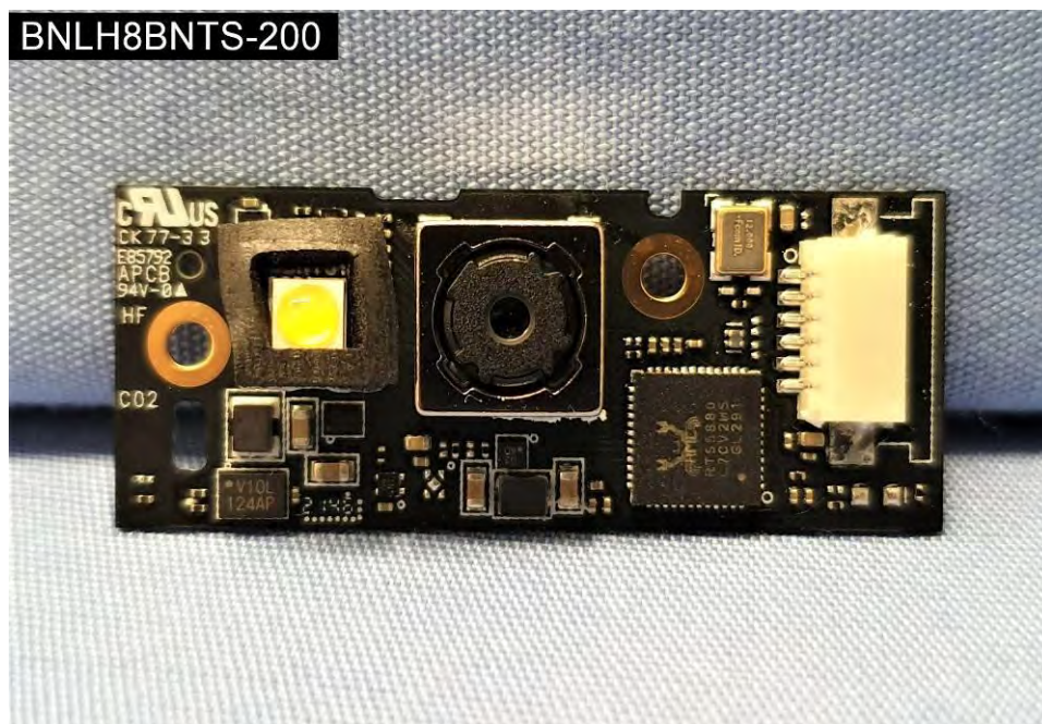
EUT Photo (50)
