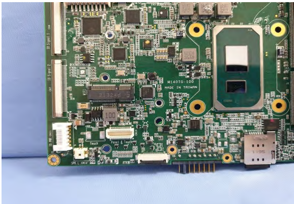
EUT Photo (54)
