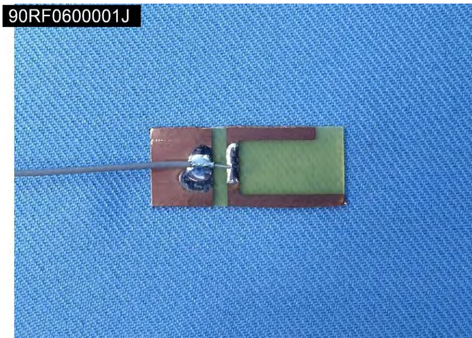
EUT Photo (12)
