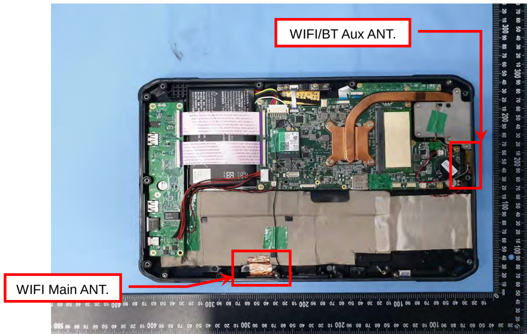
EUT Photo (6)
