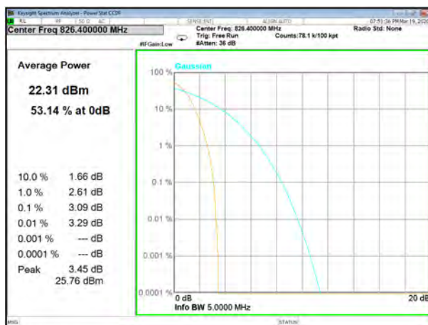
HSDPA5_Lower
