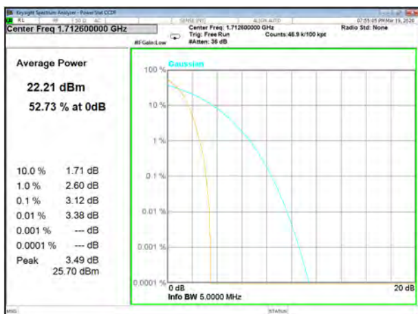
WCDMA4_Lower
