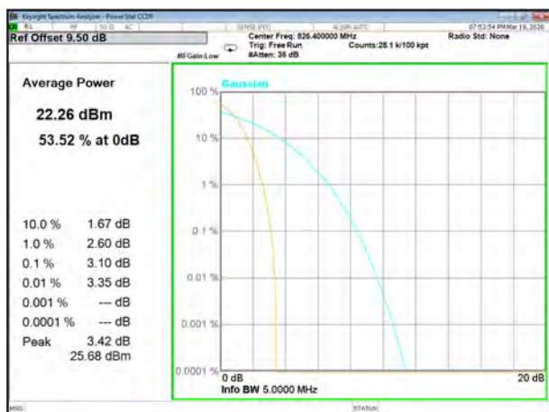
WCDMA5_Lower
