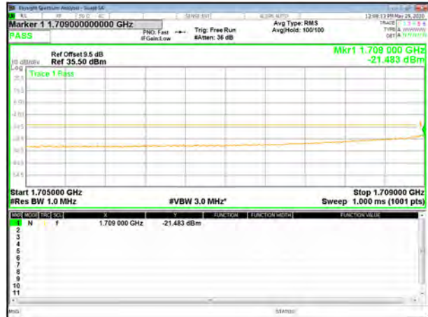
B4 WCDMA Low Band edge
