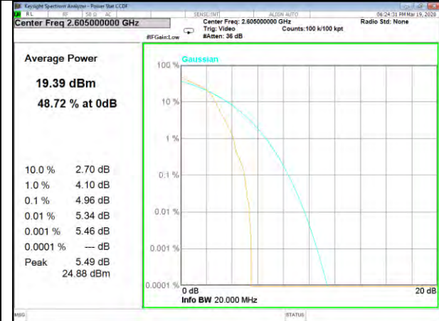
B41_1_QPSK_High
