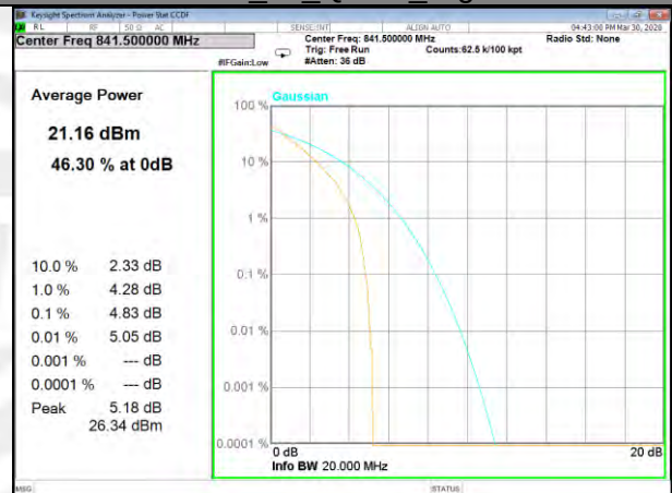
B26_50_Q16_High
