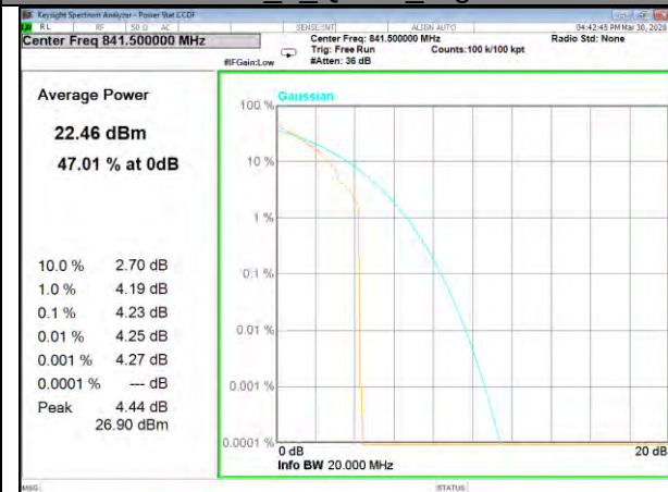
B26_1_Q16_High
