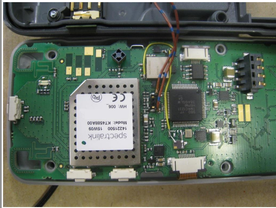
EUT 7742 PCB BOTTOM
