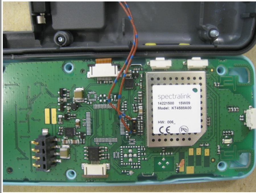
EUT 7722 PCB BOTTOM
