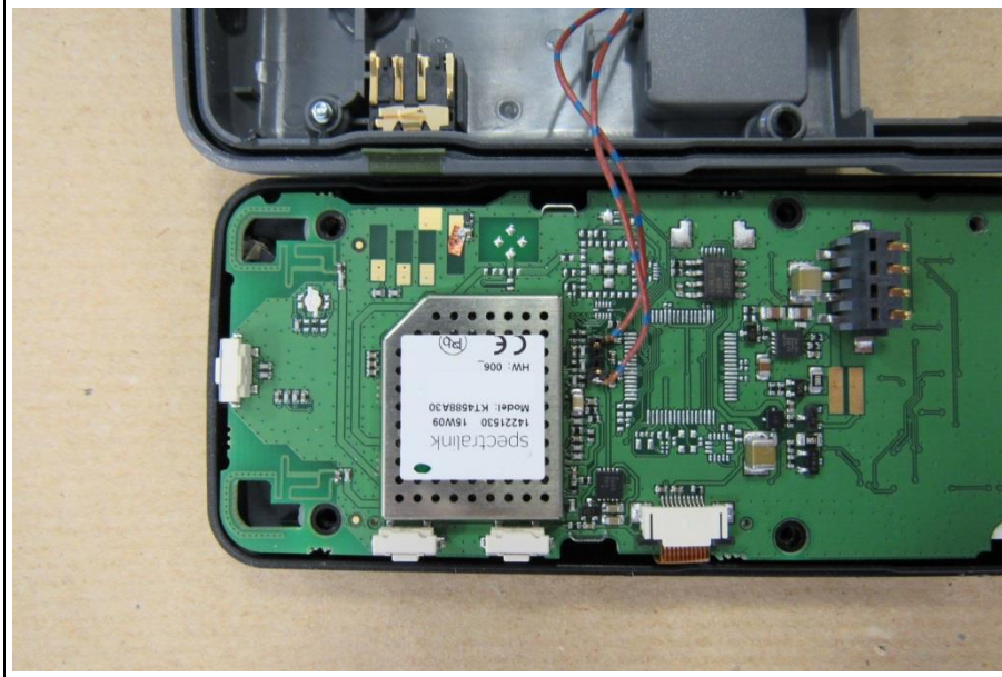
EUT 7212 PCB BOTTOM
