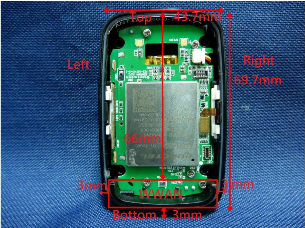
(15) EUT Photo_ DC-MD5-01
