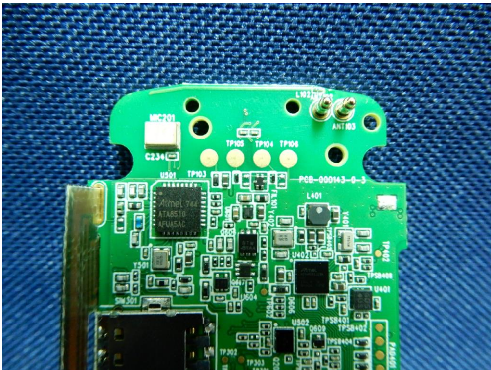
(10) EUT Photo_ DC-MD5-01
