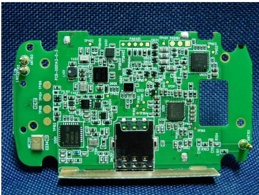
(9) EUT Photo_ DC-MD5-01
