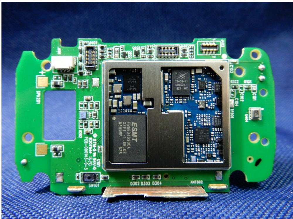
(14) EUT Photo_ DC-MD5-01
