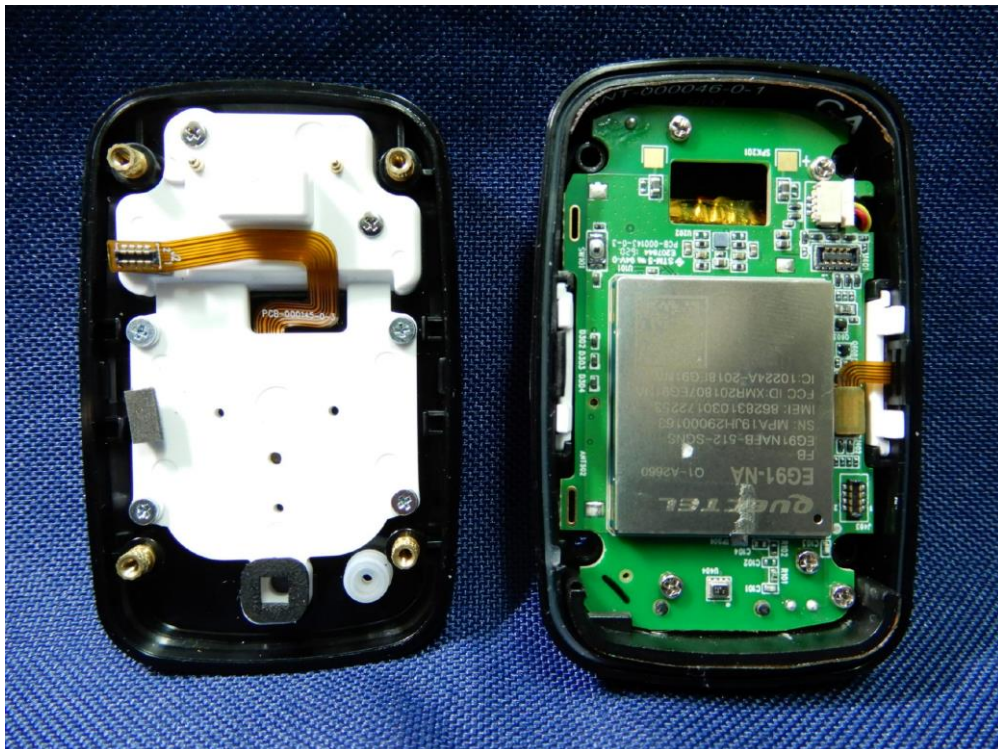
(20) EUT Photo_ DC-MD5LT-01
