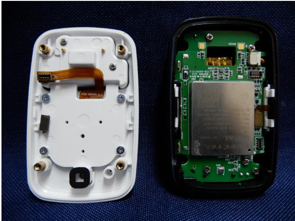
(1) EUT Photo_ DC-MD5-01
