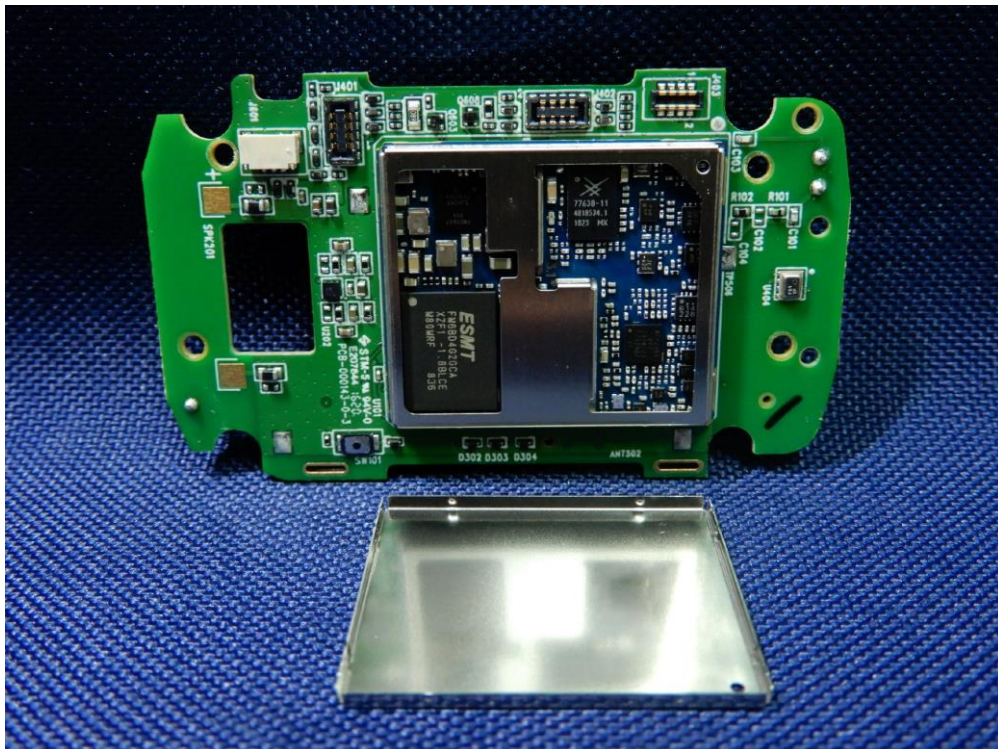
(30) EUT Photo_ DC-MD5LT-01
