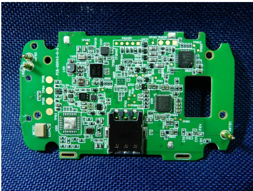
(27) EUT Photo_ DC-MD5LT-01
