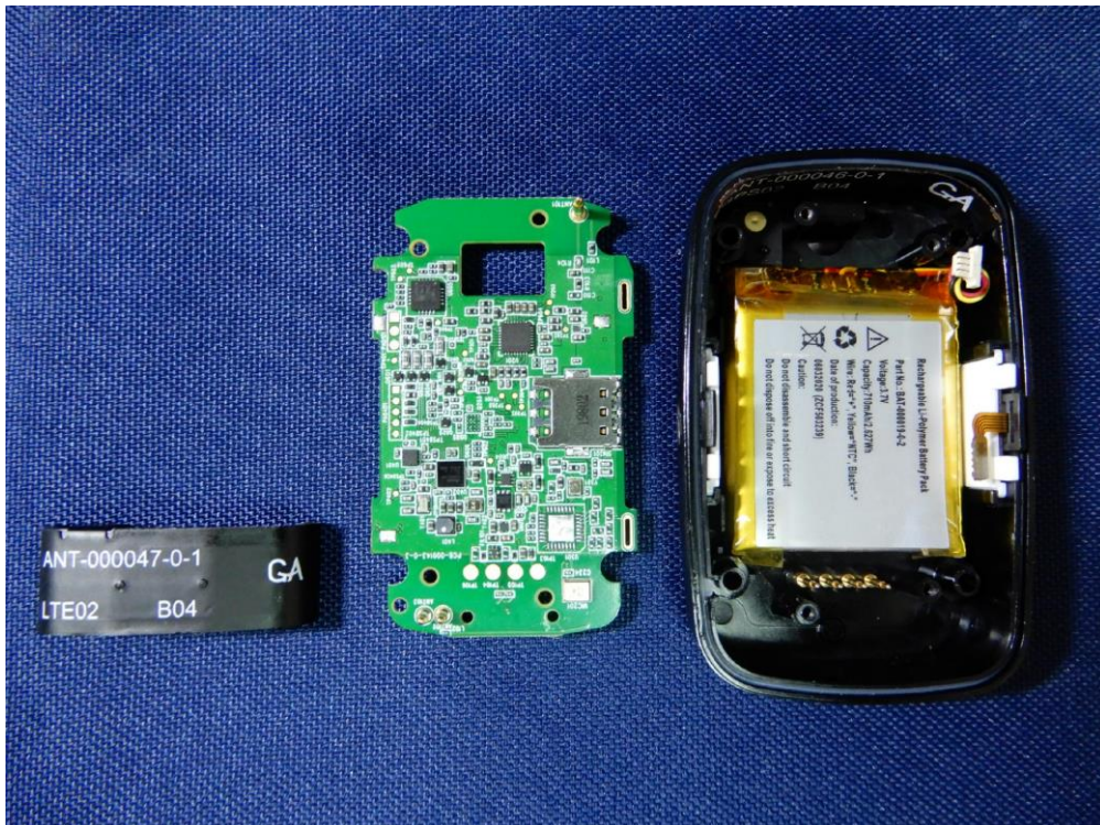
(24) EUT Photo_ DC-MD5LT-01
