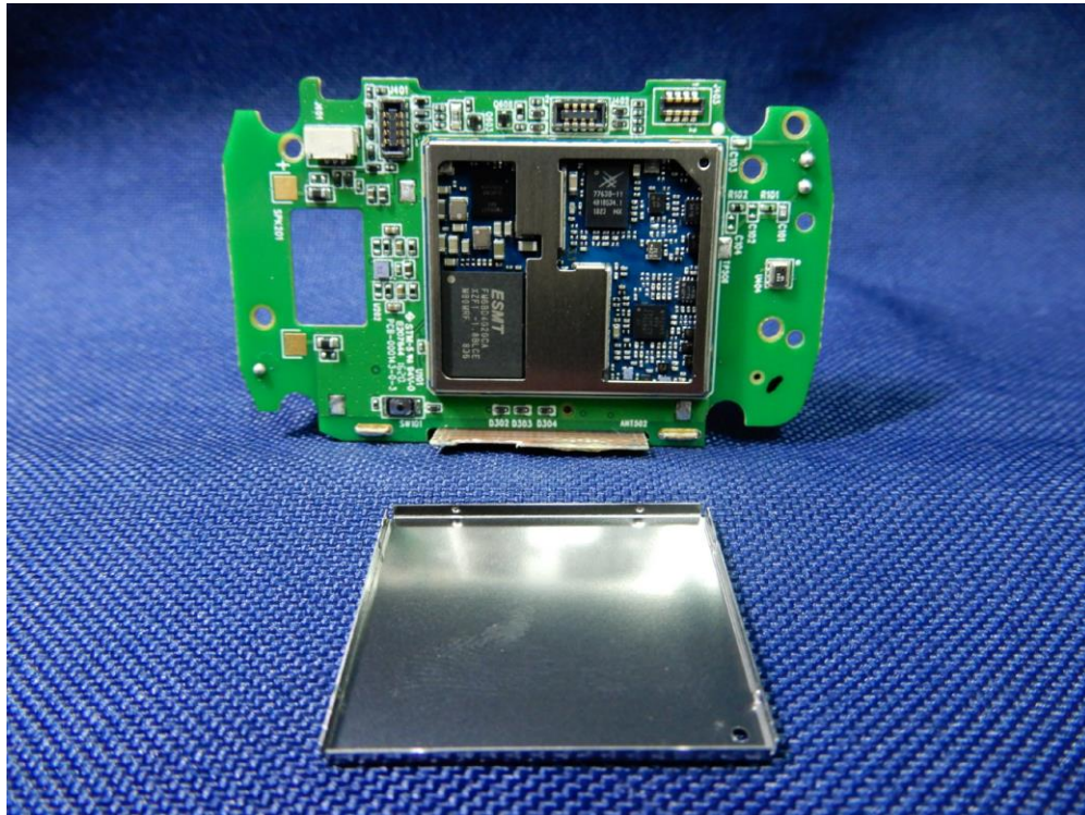
(17) EUT Photo_ DC-MD5-01
