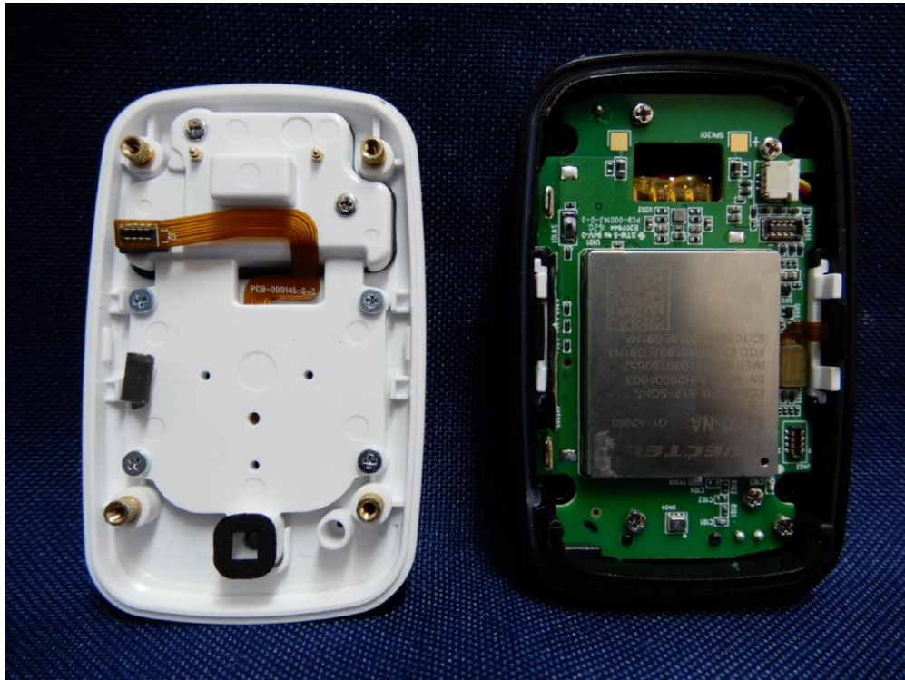
(5) EUT Photo_ DC-MD5-01
