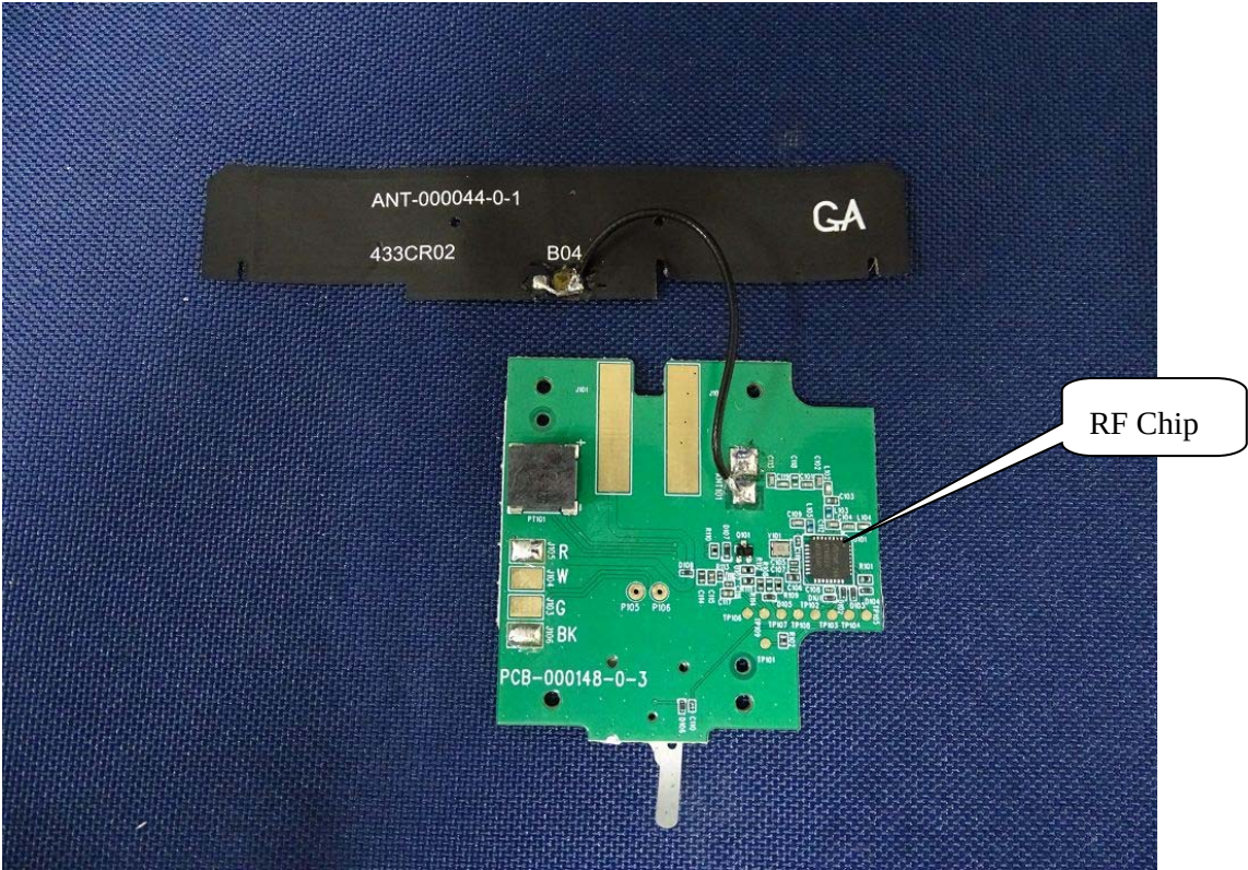
(10) EUT Photo
