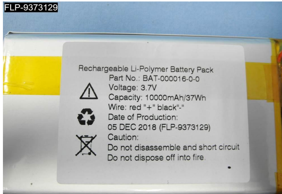
EUT Photo (36)
