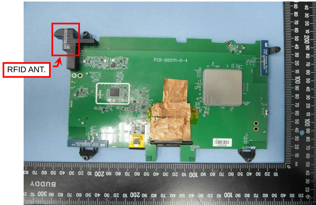
EUT Photo (4)
