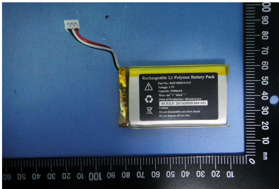
EUT Photo 22 )
