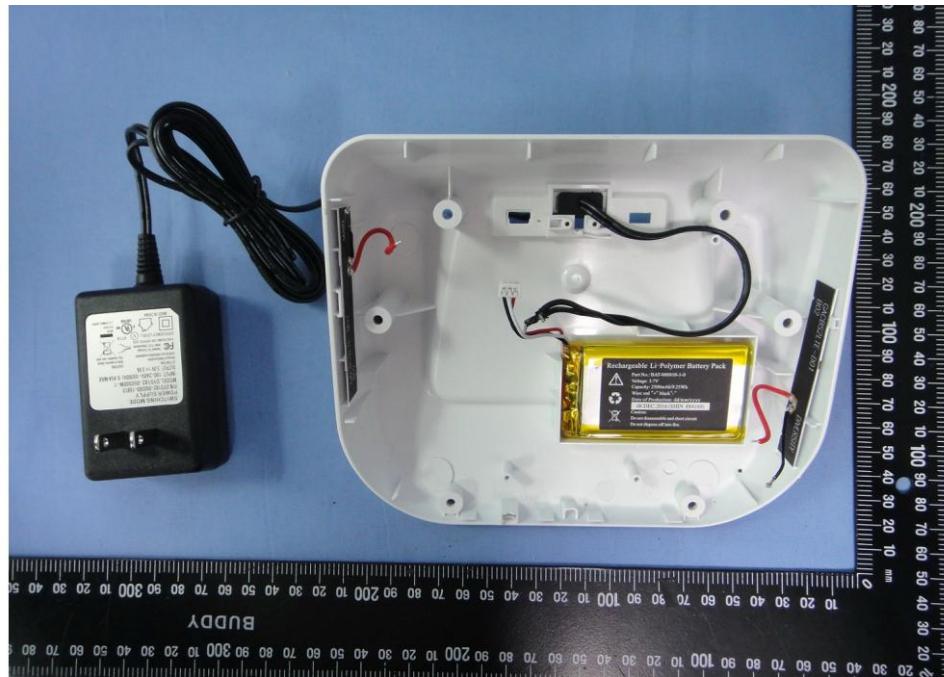
EUT Photo 22 )
