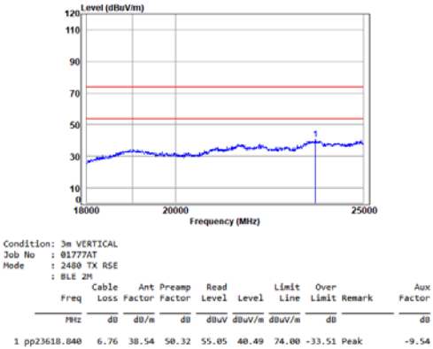
BLE_2M_TX_CH_39_Vertical
