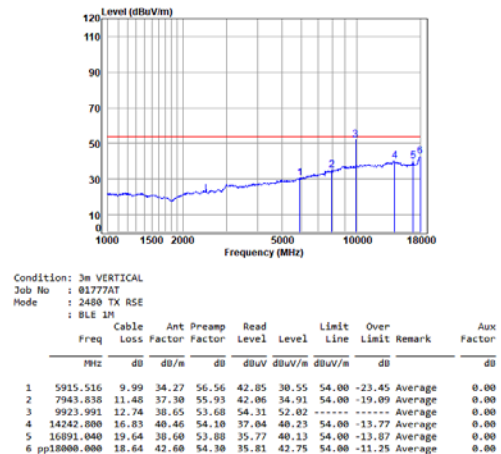
BLE_1M_TX_CH_39_Vertical-Avg
