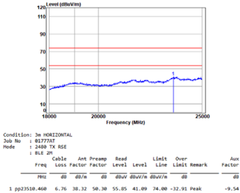
BLE_2M_TX_CH_39_Horizontal
