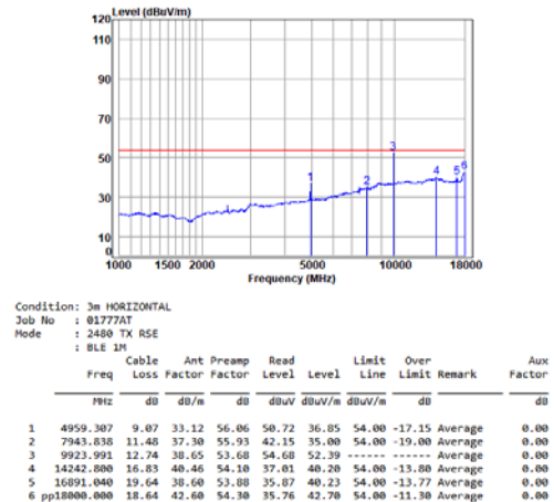
BLE_1M_TX_CH_39_Horizontal-Avg
