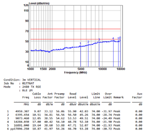
BLE_2M_TX_CH_39_Vertical
