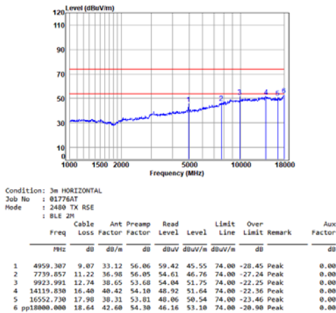
BLE_2M_TX_CH_39_Horizontal
