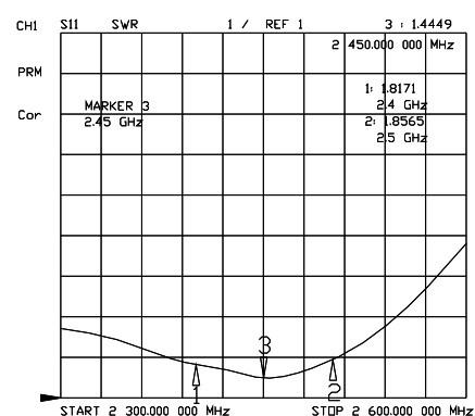
VSWR
