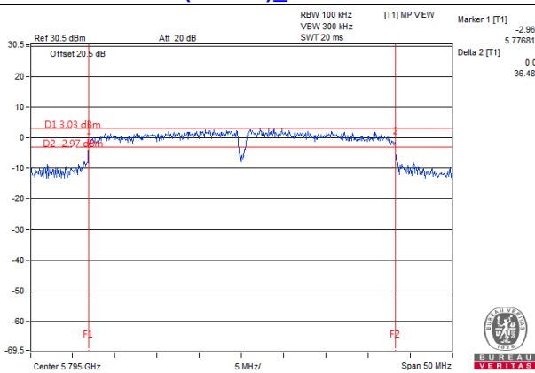
802.11n (40MHz)_Chain 0 / CH 159
