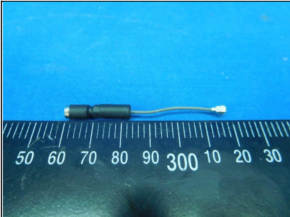
Antenna: 5GHz_Chain 1
