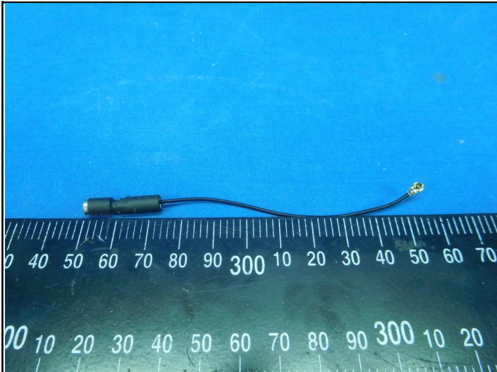
Antenna: 5GHz_Chain 3
