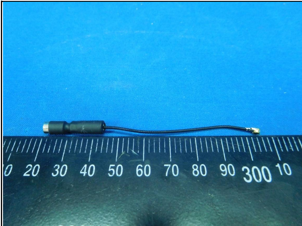
Antenna: 5GHz_Chain 2
