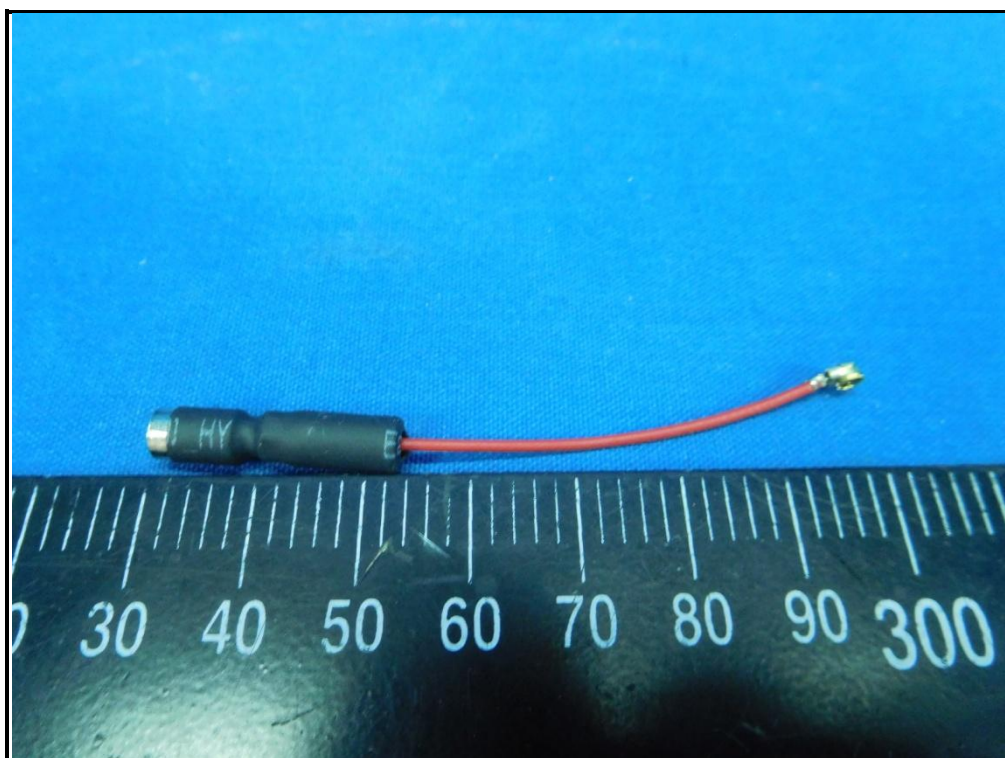
Antenna: 5GHz_Chain 0
