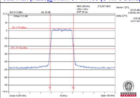
802.11ax (HE20)_Chain 3 / CH185 (U-NII-8 Band)
