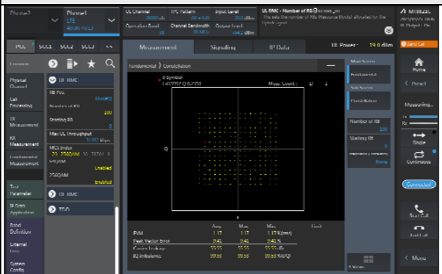
256QAM
