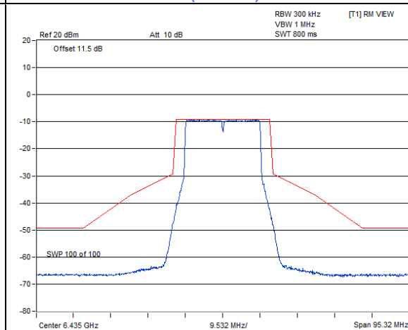
802.11be (EHT20) / Chain 0 : CH 97
