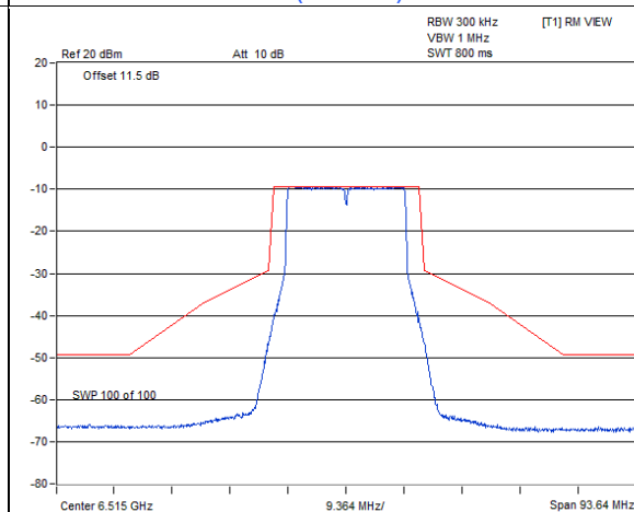
802.11be (EHT20) / Chain 0 : CH 113
