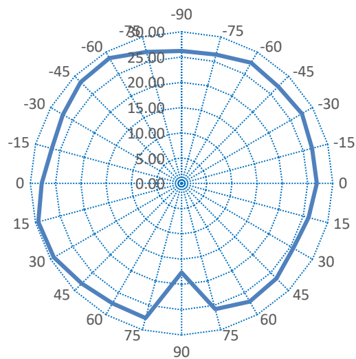
5G Ch100
