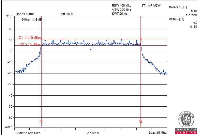
802.11a / Chain 2 : CH 177
