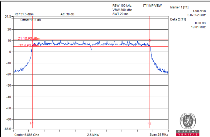
802.11be (EHT20) / Chain 3 : CH 177
