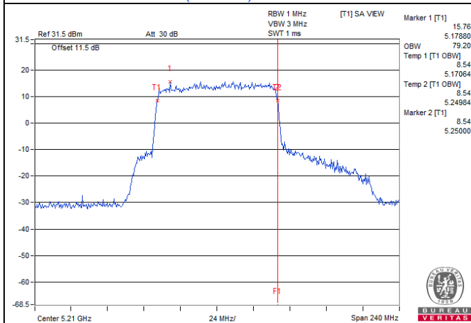
802.11be (EHT80) / Chain 2 : CH 42
