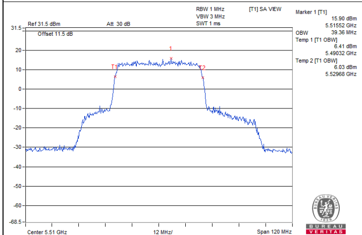
802.11be (EHT40) / Chain 0 : CH 102
