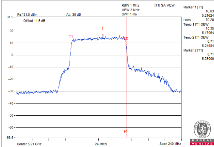
802.11be (EHT80) / Chain 0 : CH 42
