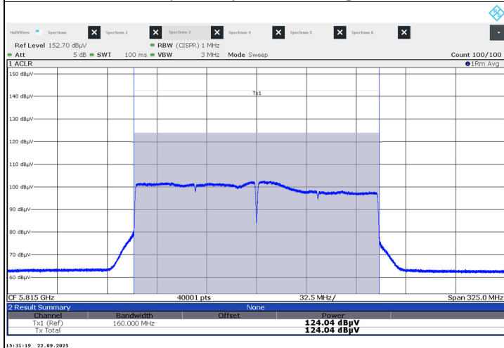
802.11be (EHT160) Beamforming: CH 163
