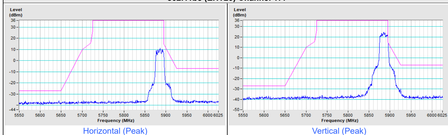
802.11be (EHT20) Channel 177
