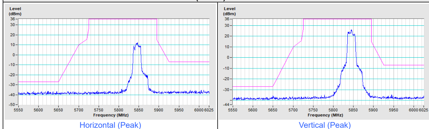
802.11be (EHT20) Channel 169
