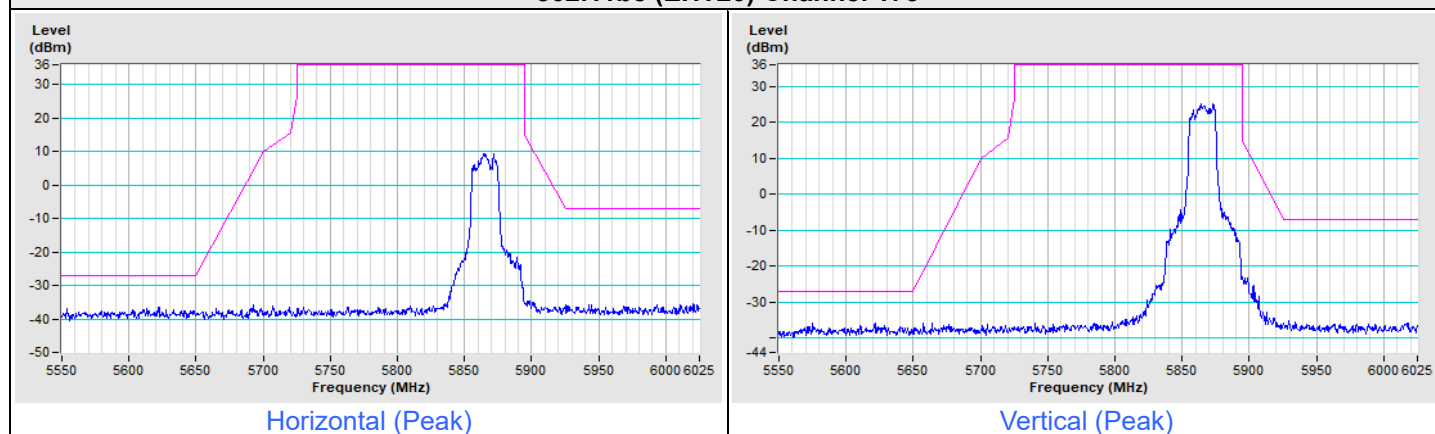
802.11be (EHT20) Channel 173
