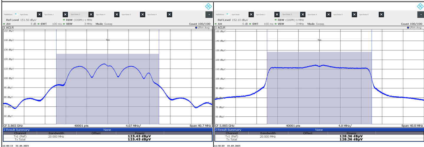
802.11a CDD: CH 173
