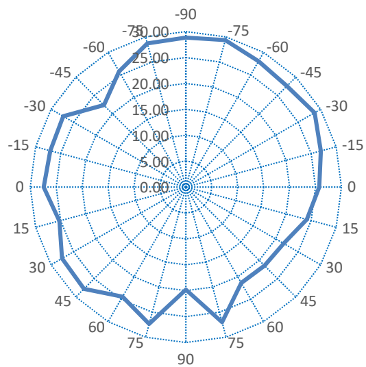
5G Ch100
