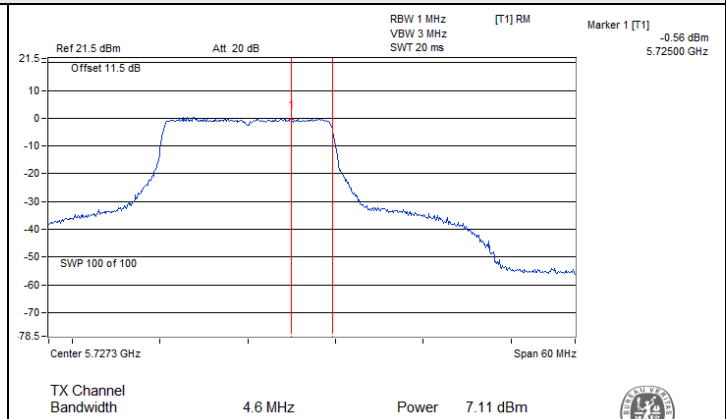
802.11be (EHT20) / Chain 0: CH 144 (U-NII-3)
