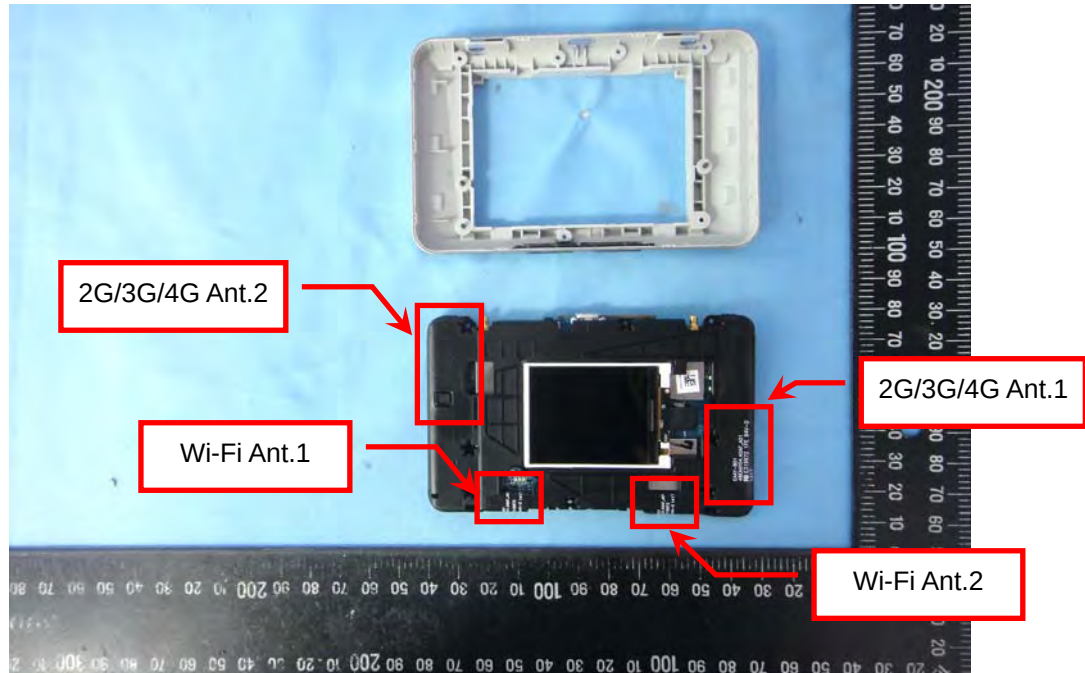
EUT Photo 7 )
