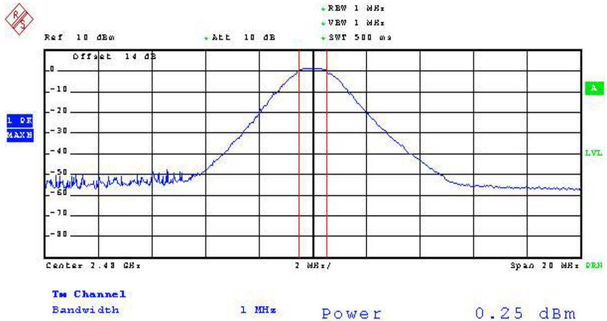
Plot3 (Channel 78) :
