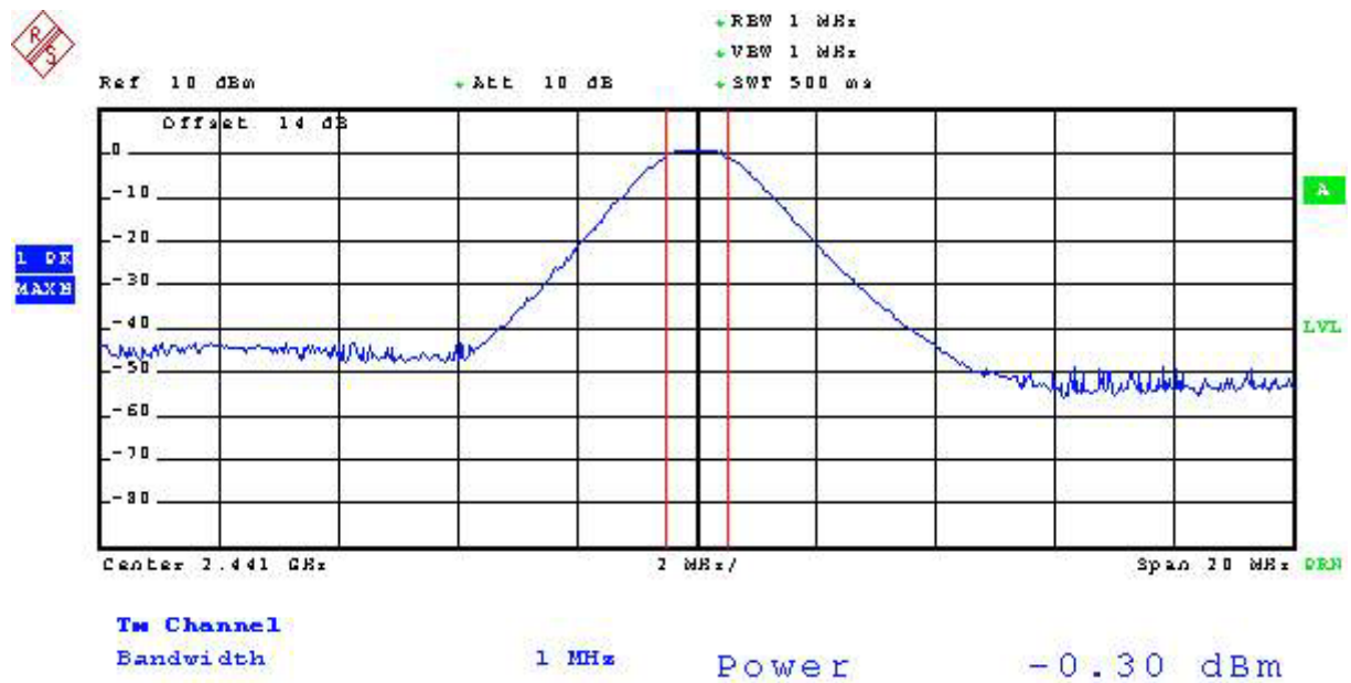
Plot2 (Channel 39) :
