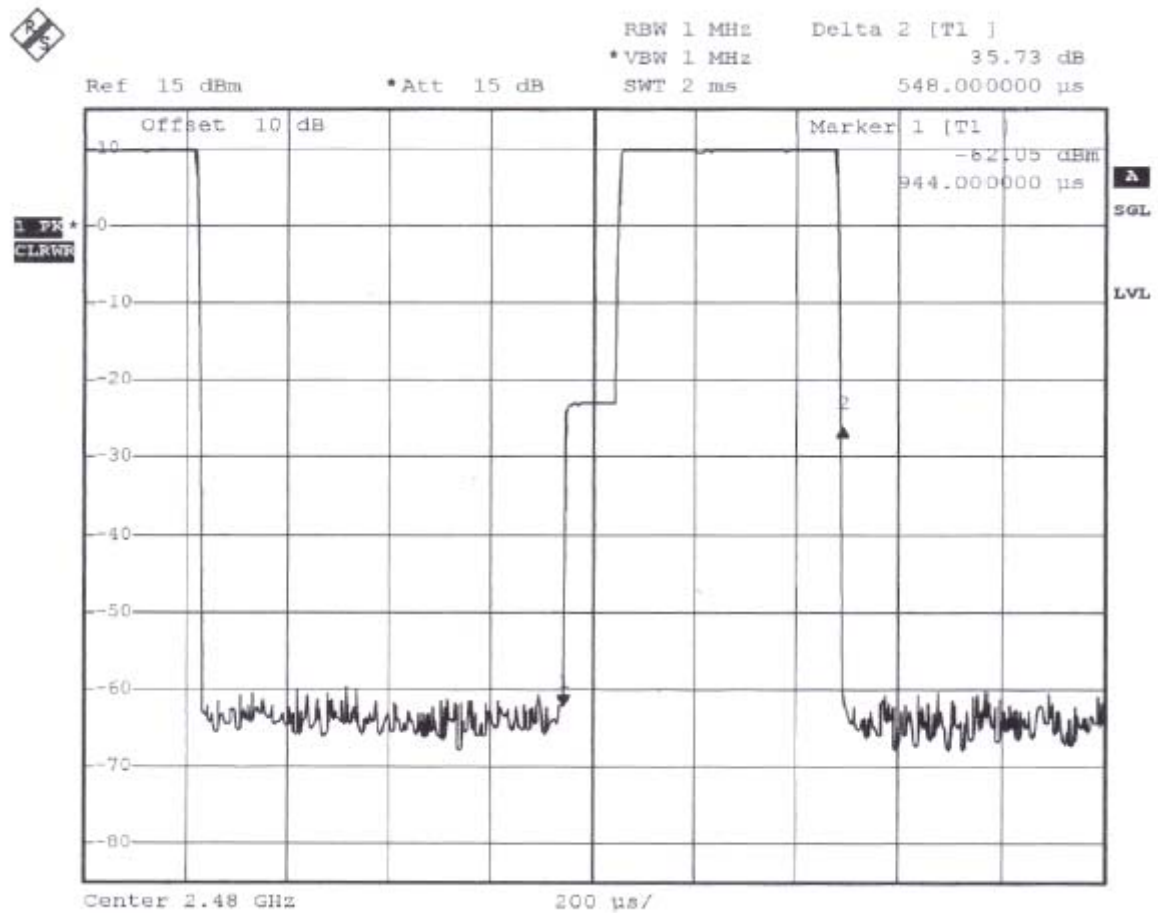
Plot3 (Channel 78) :
