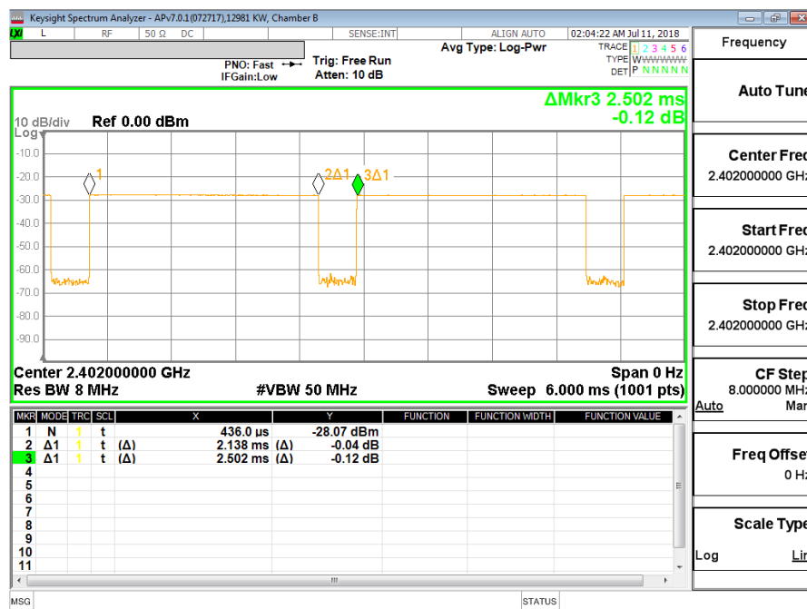
BLE (1Mbps)
