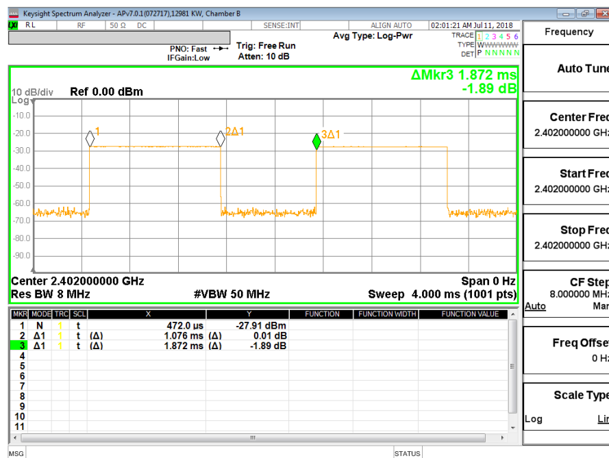
BLE (2Mbps)
