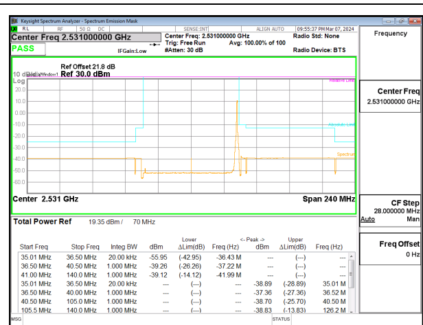
5G NR n41 70MHz QPSK Low Channel RB1-70
