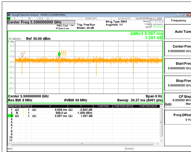
802.11be EHT20, OFDMA, 52T, 2Tx
