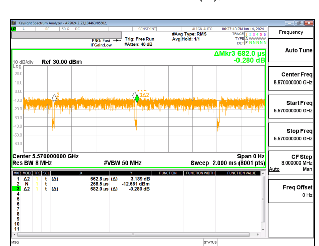
802.11be EHT160, OFDMA, 2x996T
