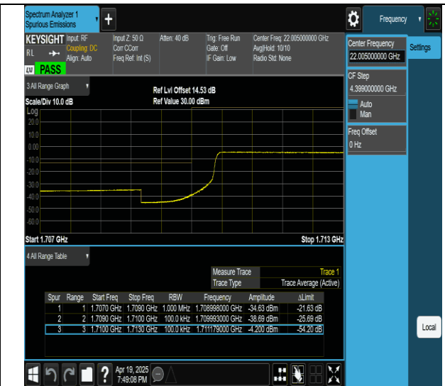
Band4-10MHz-QPSK-20000-50RB#0-PASS
