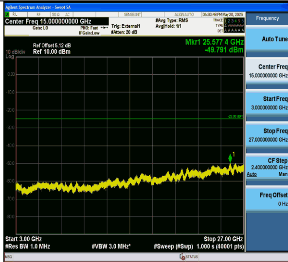
Band41-20MHz-QPSK-41490-1RB#0-3000~27000-PASS
