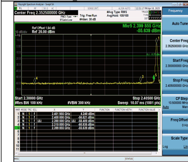
BLE 125K-Ant6-2402-PASS
