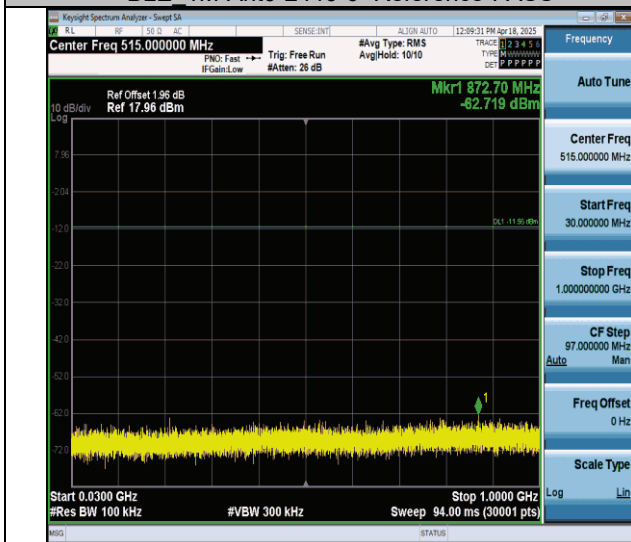
BLE 1M-Ant6-2440-30~1000-PASS
