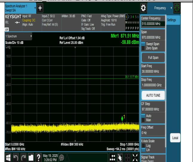
BLE 1M-Ant7-2440-30~1000-PASS
