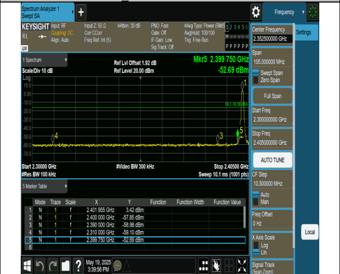
BLE 125K-Ant7-2402-PASS
