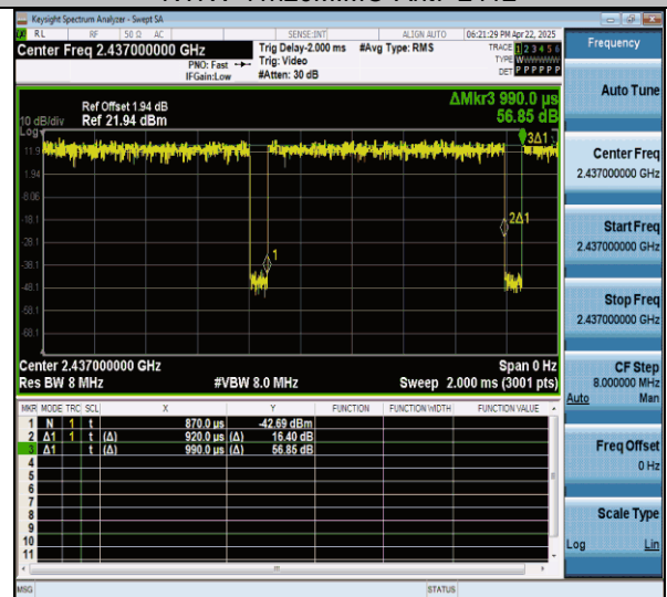
NTNV-11n20MIMO-Ant7-2437
