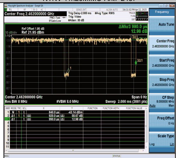
NTNV-11n20MIMO-Ant7-2462
