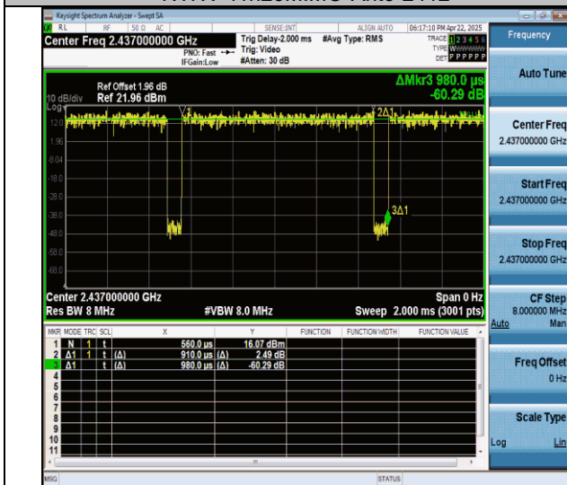
NTNV-11n20MIMO-Ant6-2437
