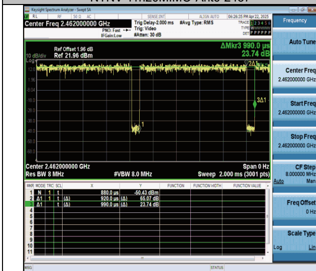
NTNV-11n20MIMO-Ant6-2462
