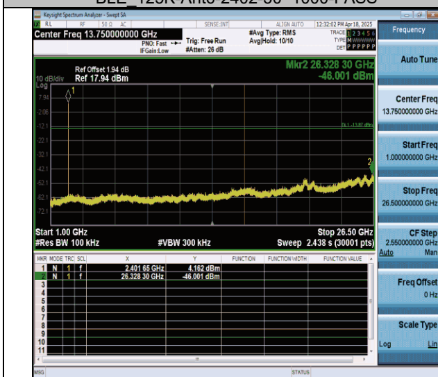
BLE 125K-Ant6-2402-1000~26500-PASS
