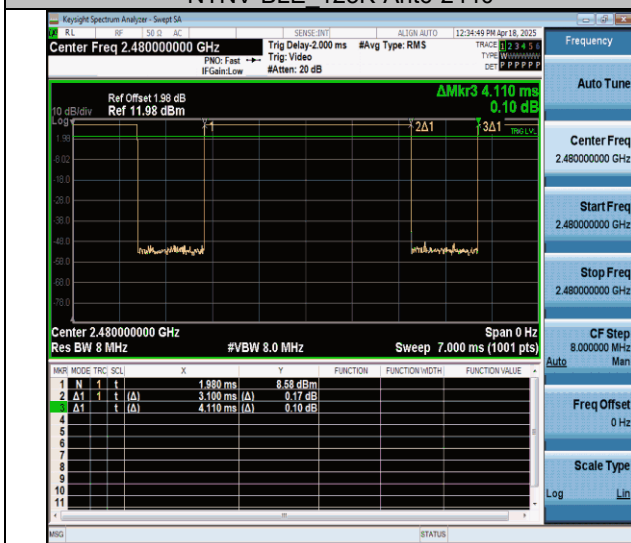
NTNV-BLE 125K-Ant6-2480
