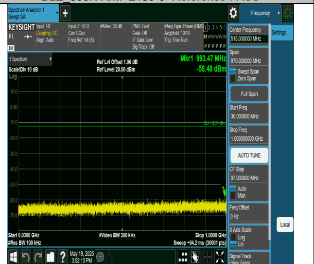
BLE 500K-Ant7-2480-30~1000-PASS
