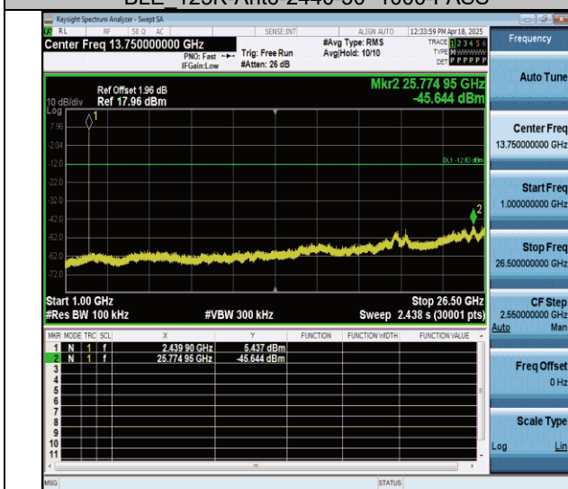
BLE 125K-Ant6-2440-1000~26500-PASS
