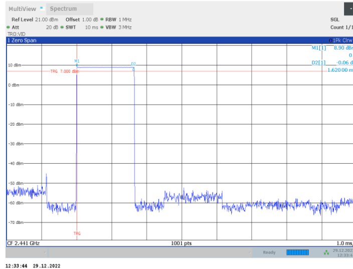
DH3_Ant6_Hop
