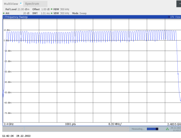
2DH5_Ant6_Hop
