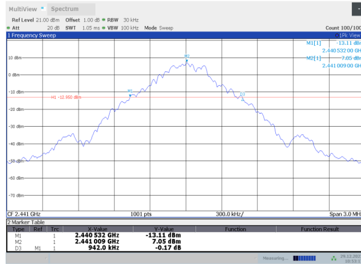
DH5_Ant6_2441
