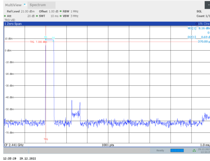
DH3_Ant6_Hop
