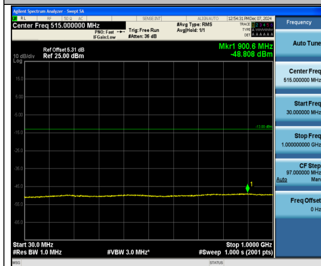
Band II-9538-30~1000MHz-PASS
