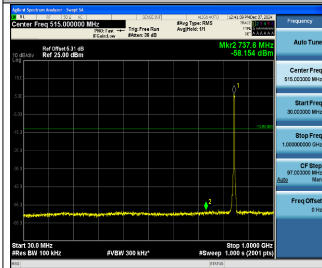
Band V-4233-30~1000MHz-PASS
