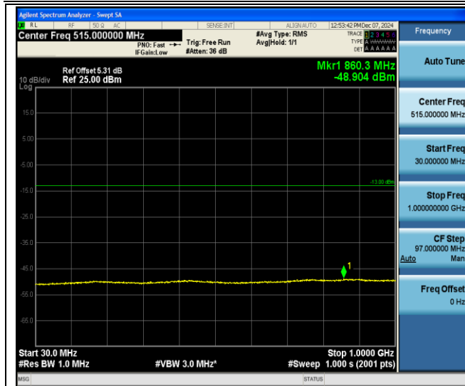
Band II-9400-30~1000MHz-PASS
