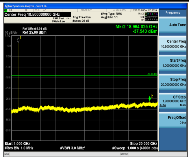
Band II-9400-1000~20000MHz-PASS
