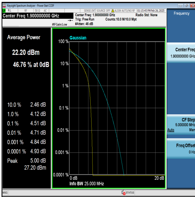
Band2-20MHz-QPSK-19100-100RB#0-PASS
