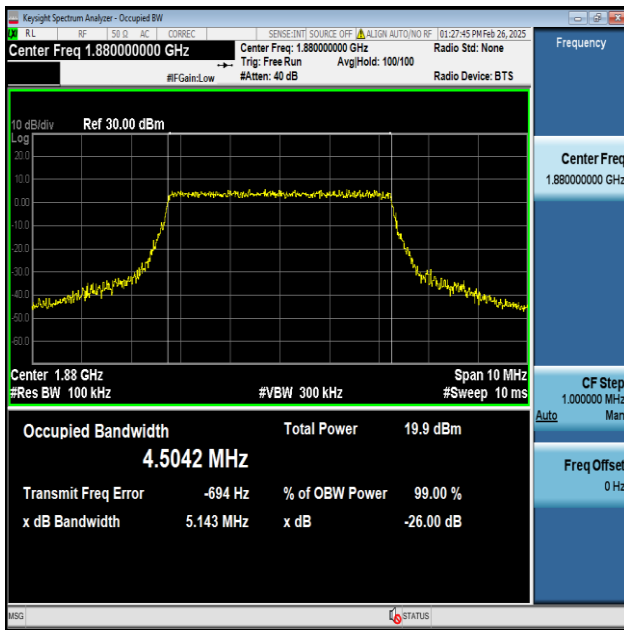
Band2-5MHz-QPSK-18900-25RB#0-PASS
