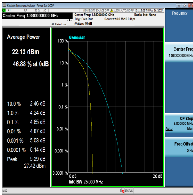
Band2-20MHz-QPSK-18900-100RB#0-PASS
