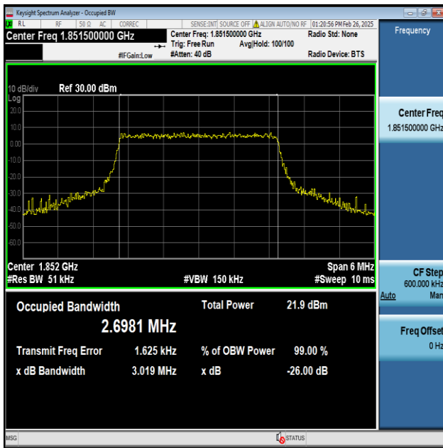
Band2-3MHz-QPSK-18615-15RB#0-PASS
