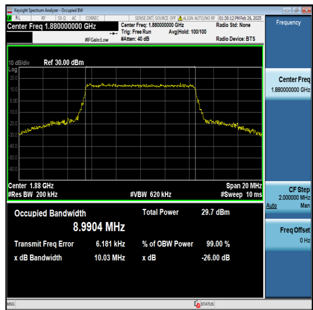
Band2-10MHz-16QAM-18900-50RB#0-PASS
