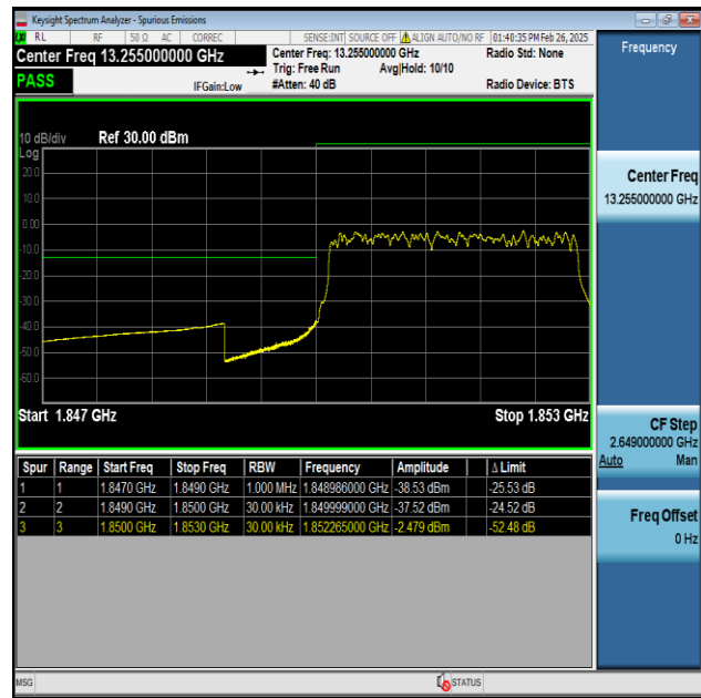
Band2-3MHz-QPSK-18615-15RB#0-PASS
