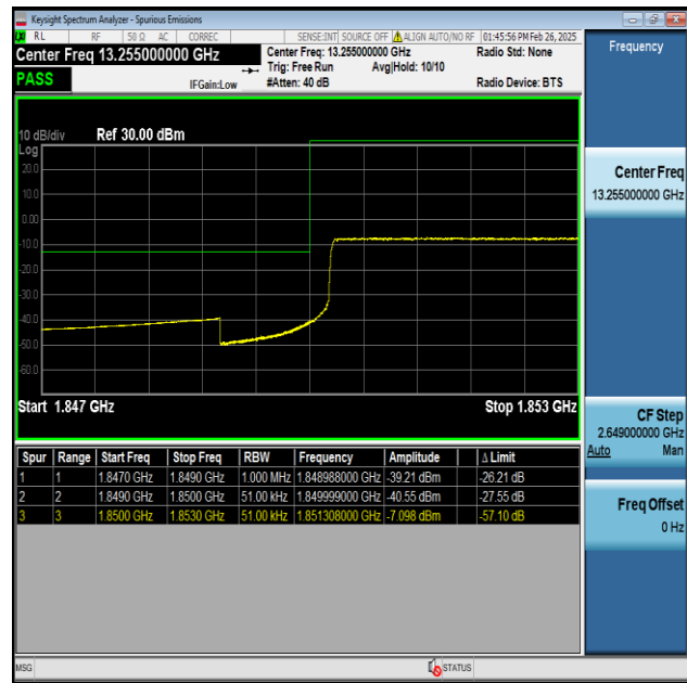
Band2-5MHz-QPSK-18625-25RB#0-PASS
