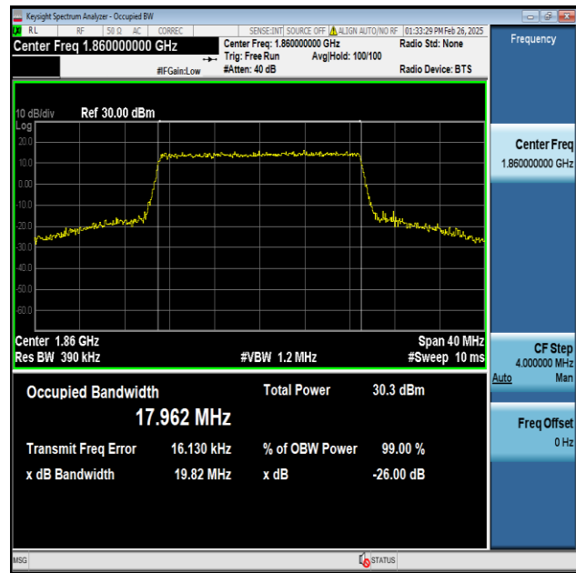
Band2-20MHz-16QAM-18700-100RB#0-PASS
