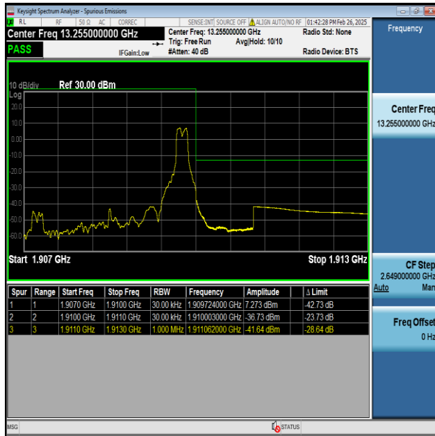
Band2-3MHz-QPSK-19185-1RB#14-PASS
