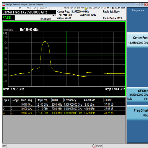
Band2-20MHz-QPSK-19100-1RB#99-PASS
