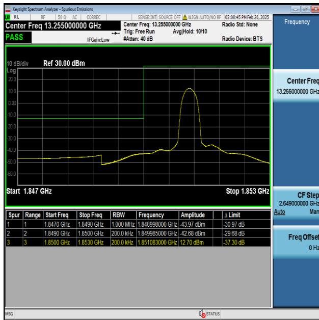
Band2-20MHz-QPSK-18700-1RB#0-PASS
