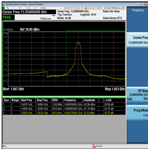
Band2-10MHz-QPSK-18650-1RB#0-PASS
