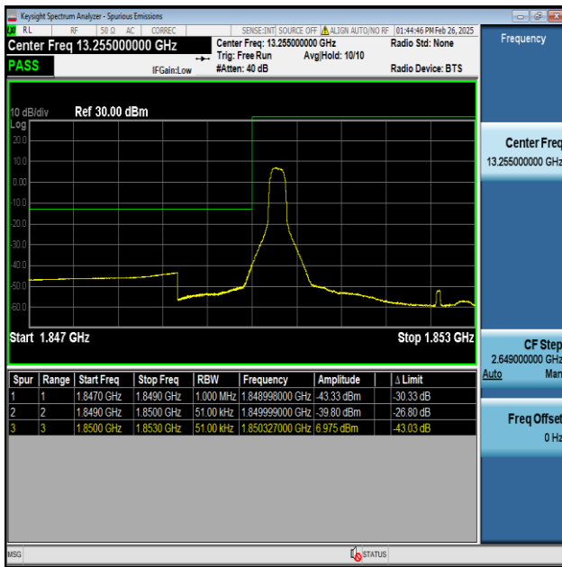
Band2-5MHz-QPSK-18625-1RB#0-PASS
