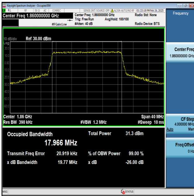
Band2-20MHz-QPSK-18700-100RB#0-PASS
