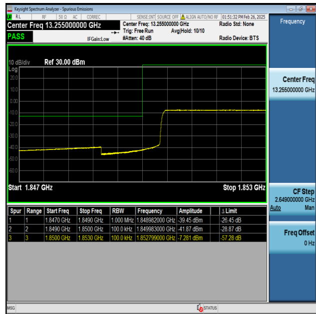
Band2-10MHz-QPSK-18650-50RB#0-PASS
