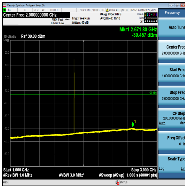
Band2-20MHz-QPSK-18900-1RB#0-1000~3000-PASS
