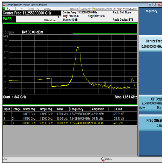
Band2-3MHz-QPSK-18615-1RB#0-PASS
