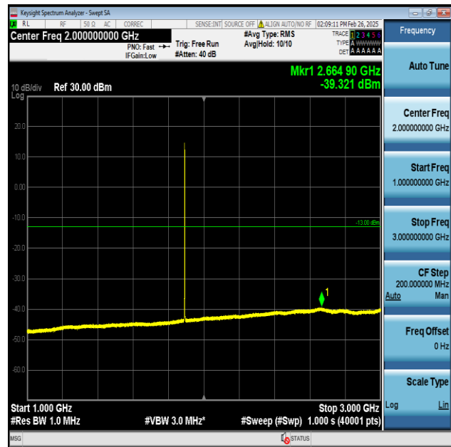
Band2-20MHz-QPSK-19100-1RB#0-1000~3000-PASS
