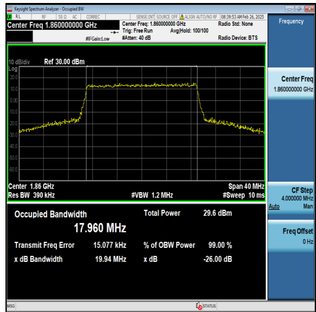
Band2-20MHz-16QAM-18700-100RB#0-PASS
