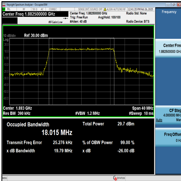
Band25-20MHz-64QAM-26365-100RB#0-PASS
