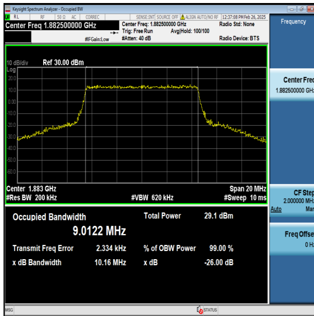
Band25-10MHz-QPSK-26365-50RB#0-PASS
