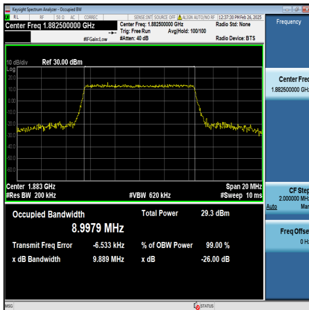
Band25-10MHz-64QAM-26365-50RB#0-PASS
