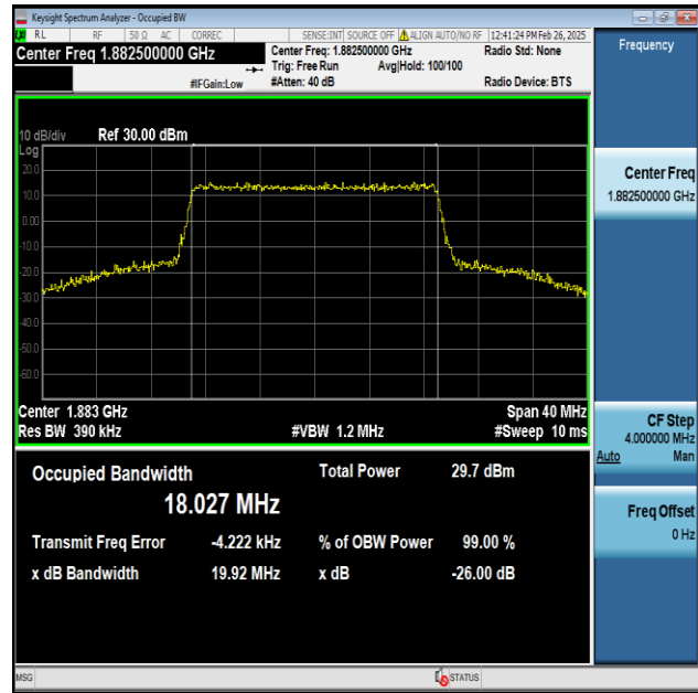
Band25-20MHz-16QAM-26365-100RB#0-PASS
