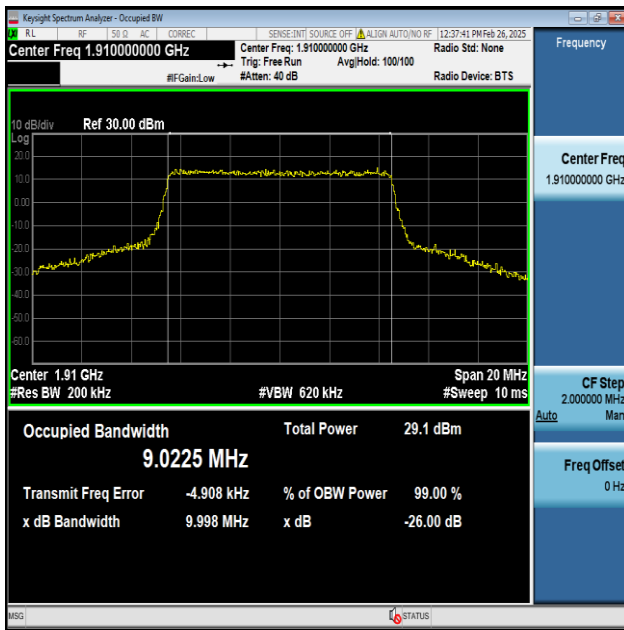
Band25-10MHz-QPSK-26640-50RB#0-PASS
