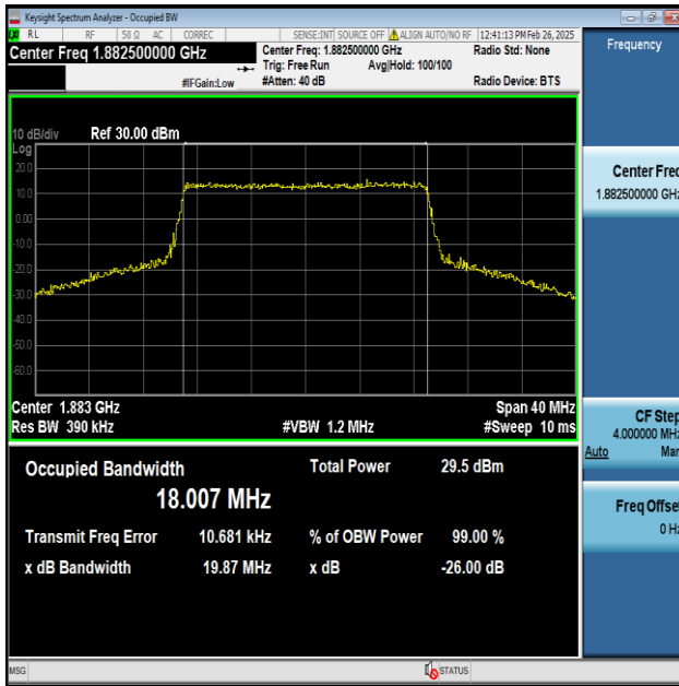
Band25-20MHz-QPSK-26365-100RB#0-PASS
