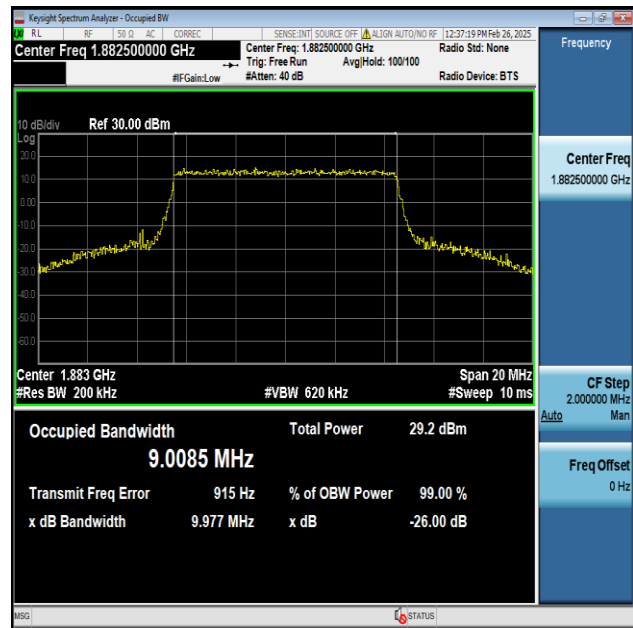
Band25-10MHz-16QAM-26365-50RB#0-PASS
